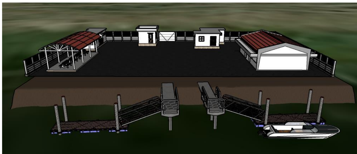
Figure 39: Embarcadère du type B : pontons flottants
